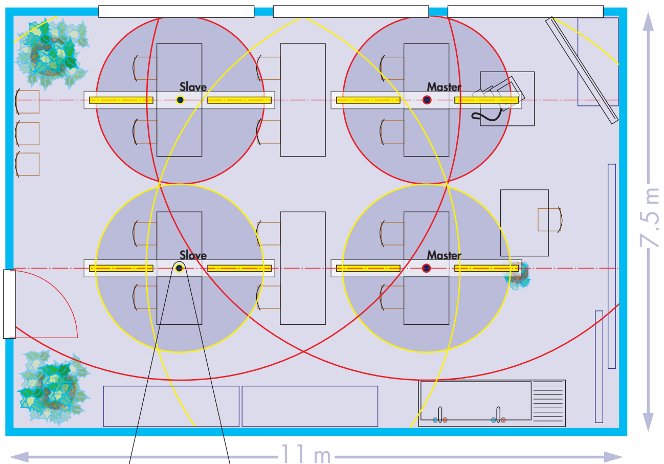
Montage in Pendelleuchte PD9
