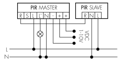
Master-Slave-Betrieb
