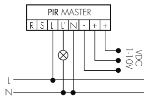
Master-Master-Betrieb
