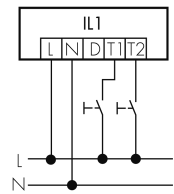
Normalbetrieb mit externem Taster
