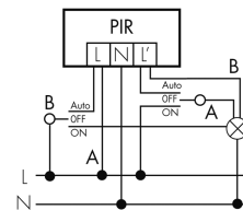
Betrieb mit Drehschalter «Hand - 0 - Automat»
