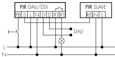
Master-Slave-Betrieb mit externem Taster
