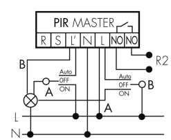
Fonctionnement avec interrupteur rotatif «Manuel - 0 - Automatique»
