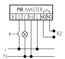
Fonctionnement normal avec bouton externe
