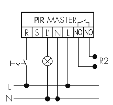
Fonctionnement Master-Slave
