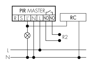
Fonctionnement normal avec circuit RC
