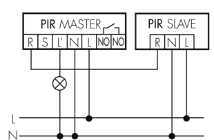
Fonctionnement normal avec bouton externe
