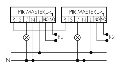
Fonctionnement normal avec circuit RC
