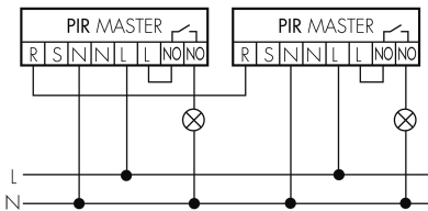
Fonctionnement Master-Master
