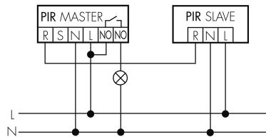
Fonctionnement Master-Slave
