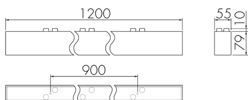
Dimensions en mm
