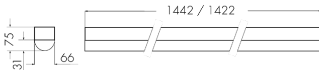
Dimensions en mm
