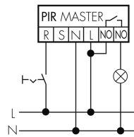
Fonctionnement Master-Slave
