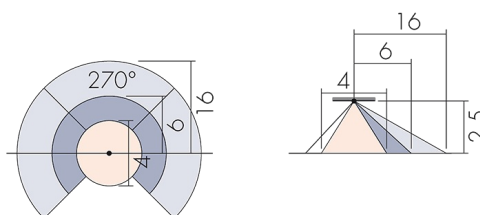
Dimensioni in m
