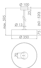
Dimensioni in mm
