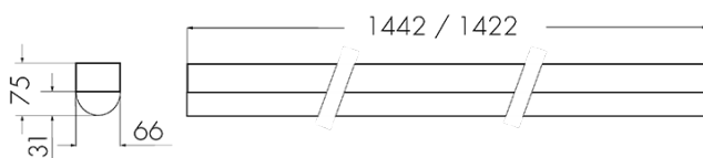
Dimensioni in mm
