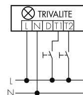
Funzionamento normale con tasto esterno
