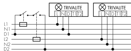
Funzionamento gruppi/Funzionamento sistema attraverso 2 gruppi fusibili
