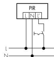
Dauerlichtbetrieb mit externem Schalter
