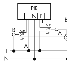
Betrieb mit Drehschalter «Hand - 0 - Automat»
