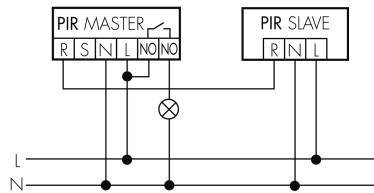
Master-Slave-Betrieb
