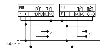
Master-Master-Betrieb
