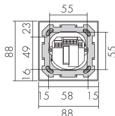
Vue arrière
