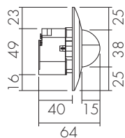
Vue latérale
